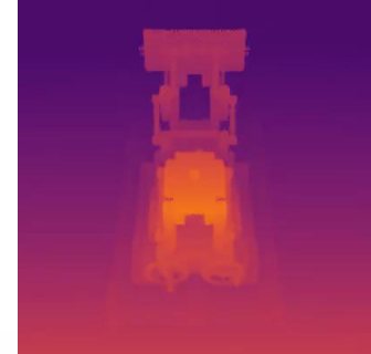
ref. NeRF
