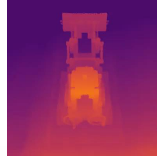
ref. NeRF
